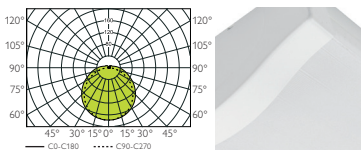
POLY T8 2x36W OPAL
