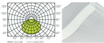
POLY T8 2x36W PRISMA
