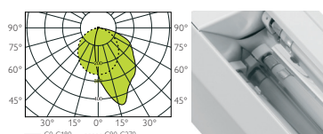
BASIC ASYM SU 1x54W
