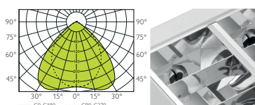
BASIC II 1x2L SU T5 1x28W PML
