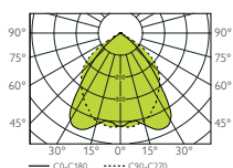
BASIC II 1x2L SU T5 4x14W PSL MIRO4
